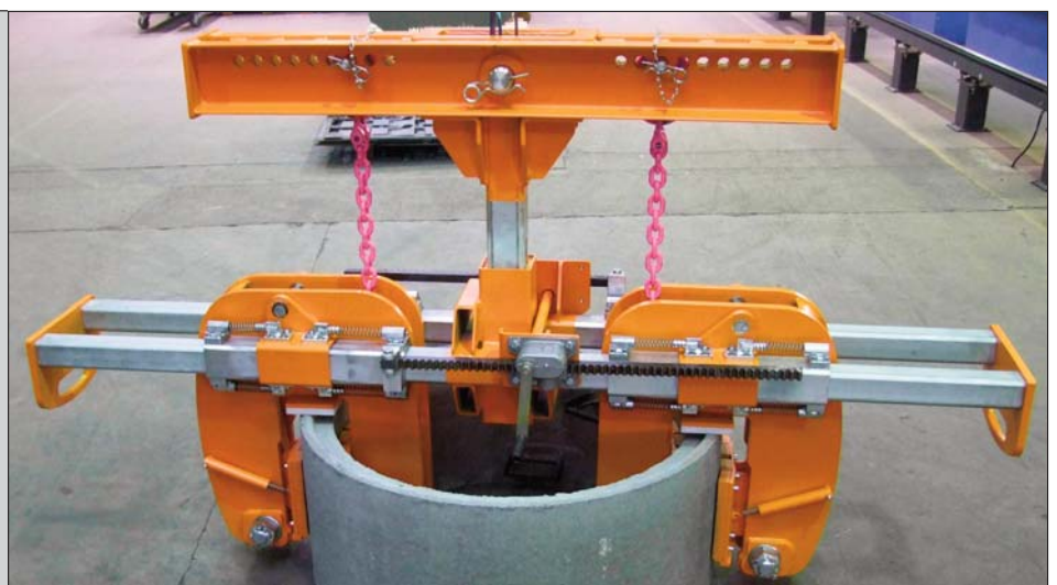
Rohrgreifer RG 10 mit gleichzeitiger, stufenloser Einstellung auf die Nennweite über Zahnstangenwinde
